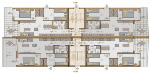
BENE ZGRADE MEDULIN ZGRADA A + B TLOCRT 2. KAT.
